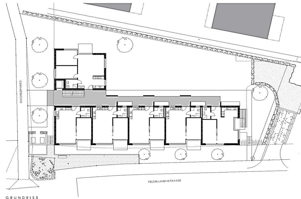
GRUNDRISS
